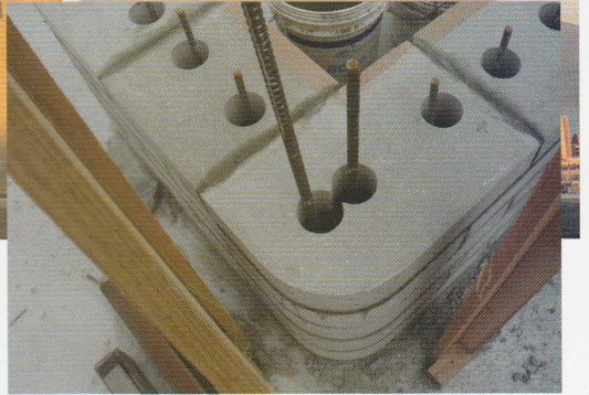
南九州一帯に堆積する火砕流堆積物の「シラス」を素材にしたシラスブロックを構造材として使用。
