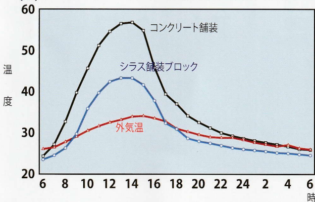
(℃) シラスブロックによる舗装面温度抑制効果
